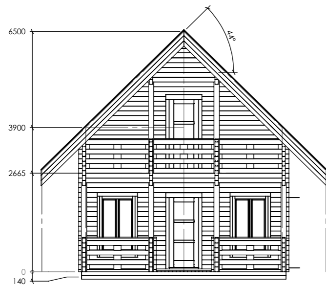
Facade A-D
