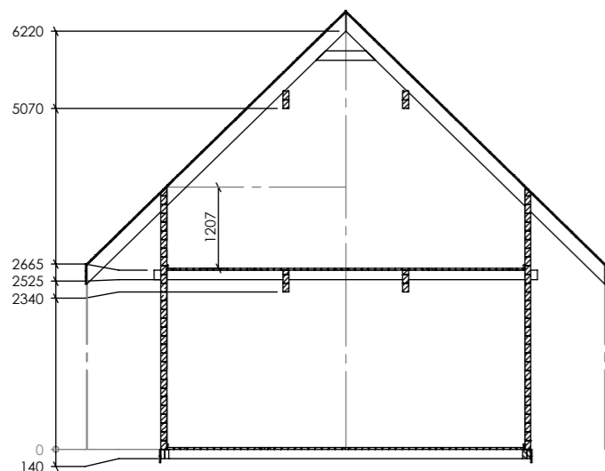
A-A
